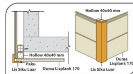
b. Outside corner menggunakan Lis Siku Luar
