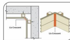
b. Inside Corner menggunakan Lis Crescent
