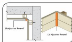
a. Inside Corner menggunakan Lis Quarter Round
