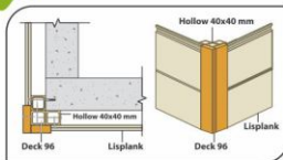
a. Outside corner menggunakan Deck 96
